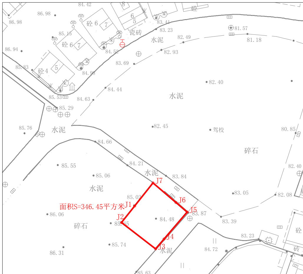
深圳市深能燃气有限公司同胜供应站平面图
