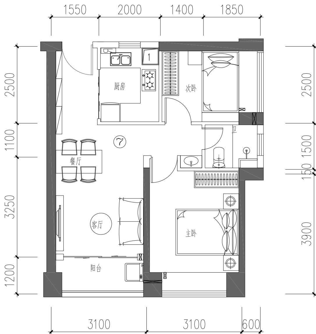
06/07户型平面图
