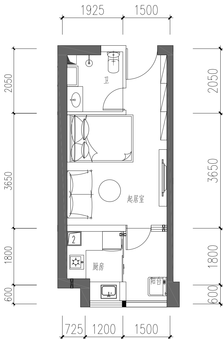
09/12户型平面图
