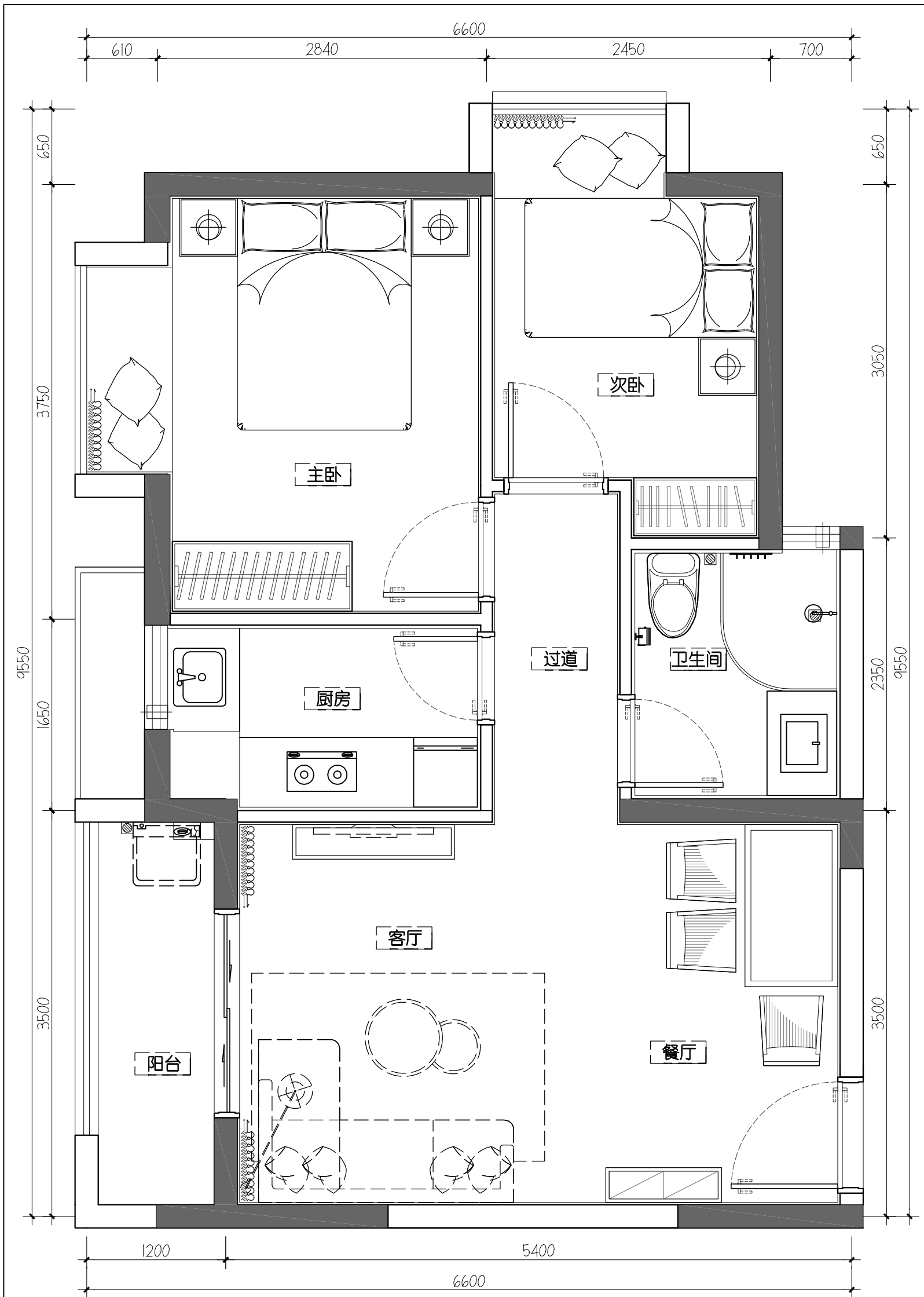
K1/K2户型平面图 两房面积约65m 2
