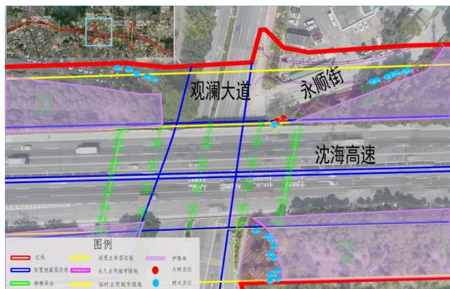
图 5 观澜大道段平面图
