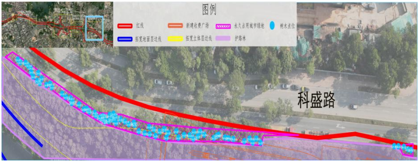
图 3 五和大道段平面图
