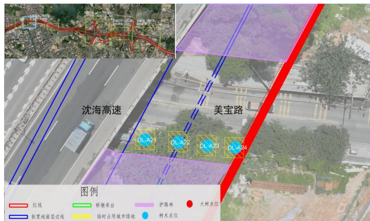
图 11 美宝路段平面图
