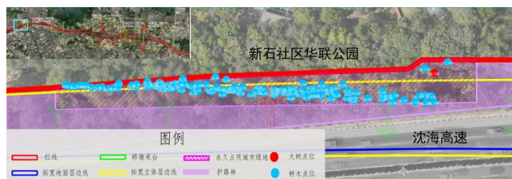
图 13 新石社区华联公园段平面图
