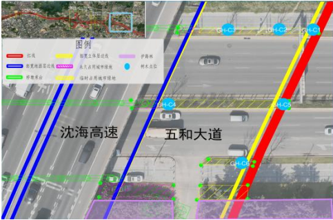
图 2 五和大道段平面图
