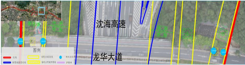
图 4 龙华大道段平面图
