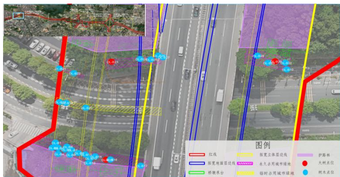
图 12 华荣路段平面图
