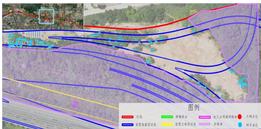
图 6 茜坑老村段平面图
