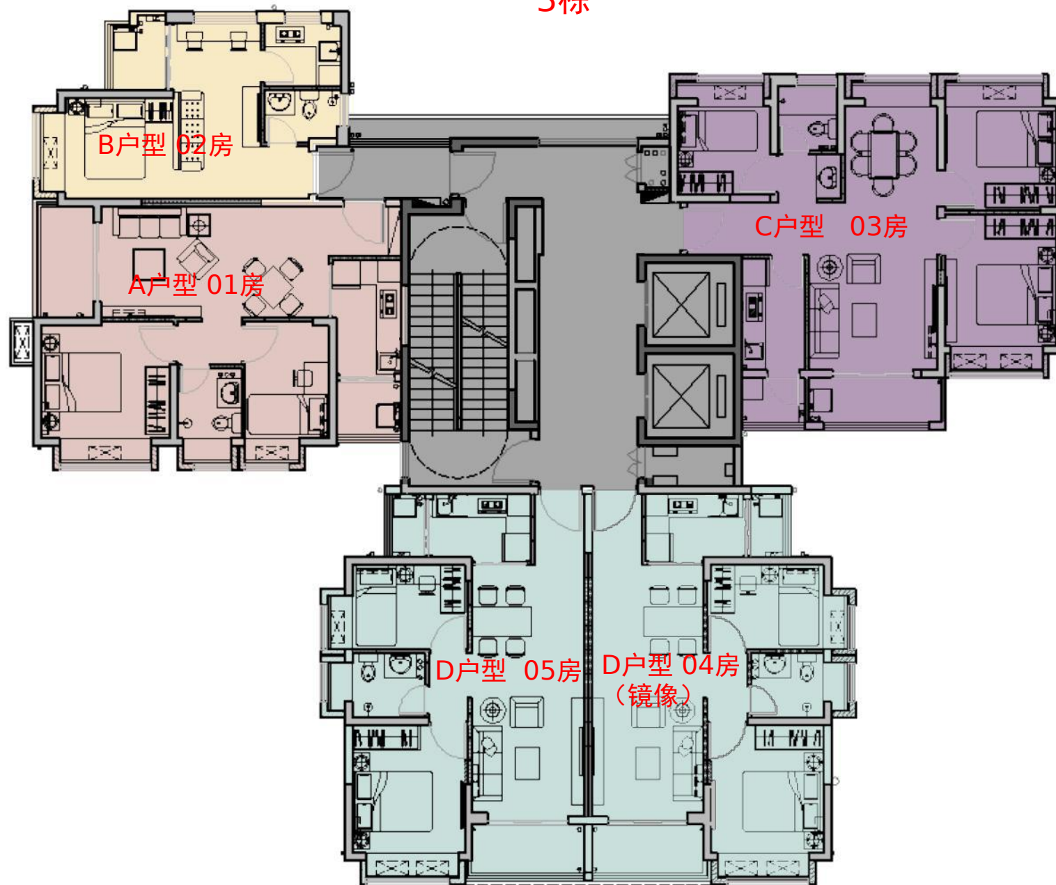
3栋2~34层平面图
