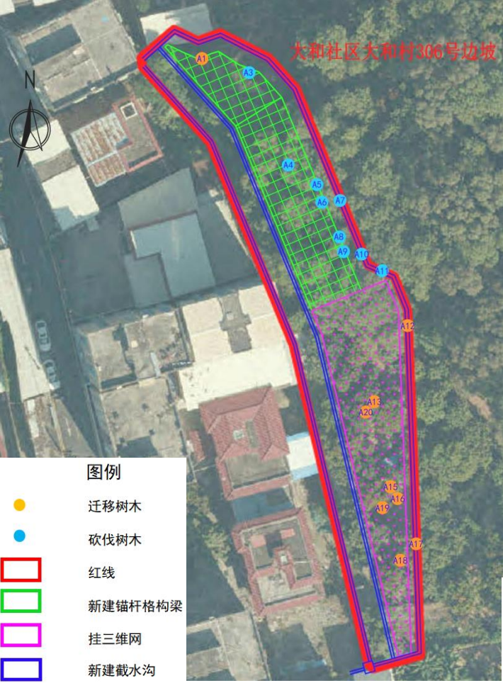
大和社区大和村 306 号边坡航拍点位图
