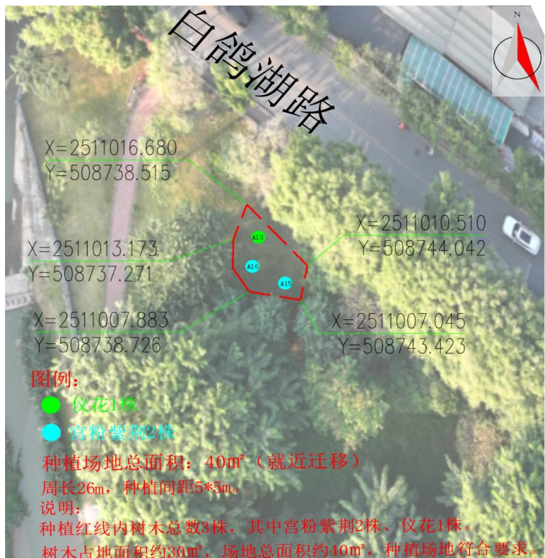
种植场地布局图
