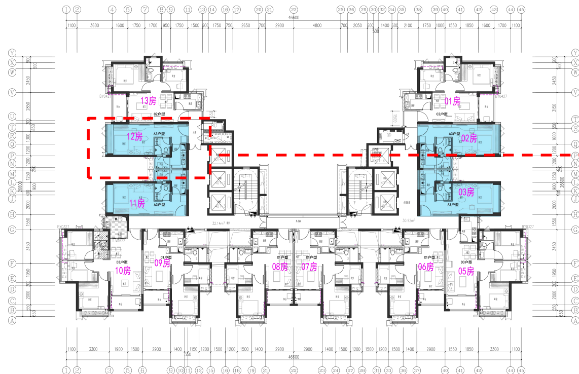
标准层平面图
