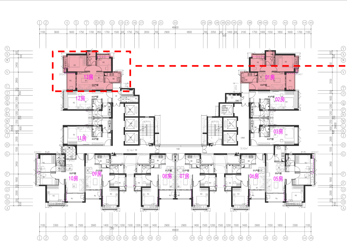
标准层平面图
