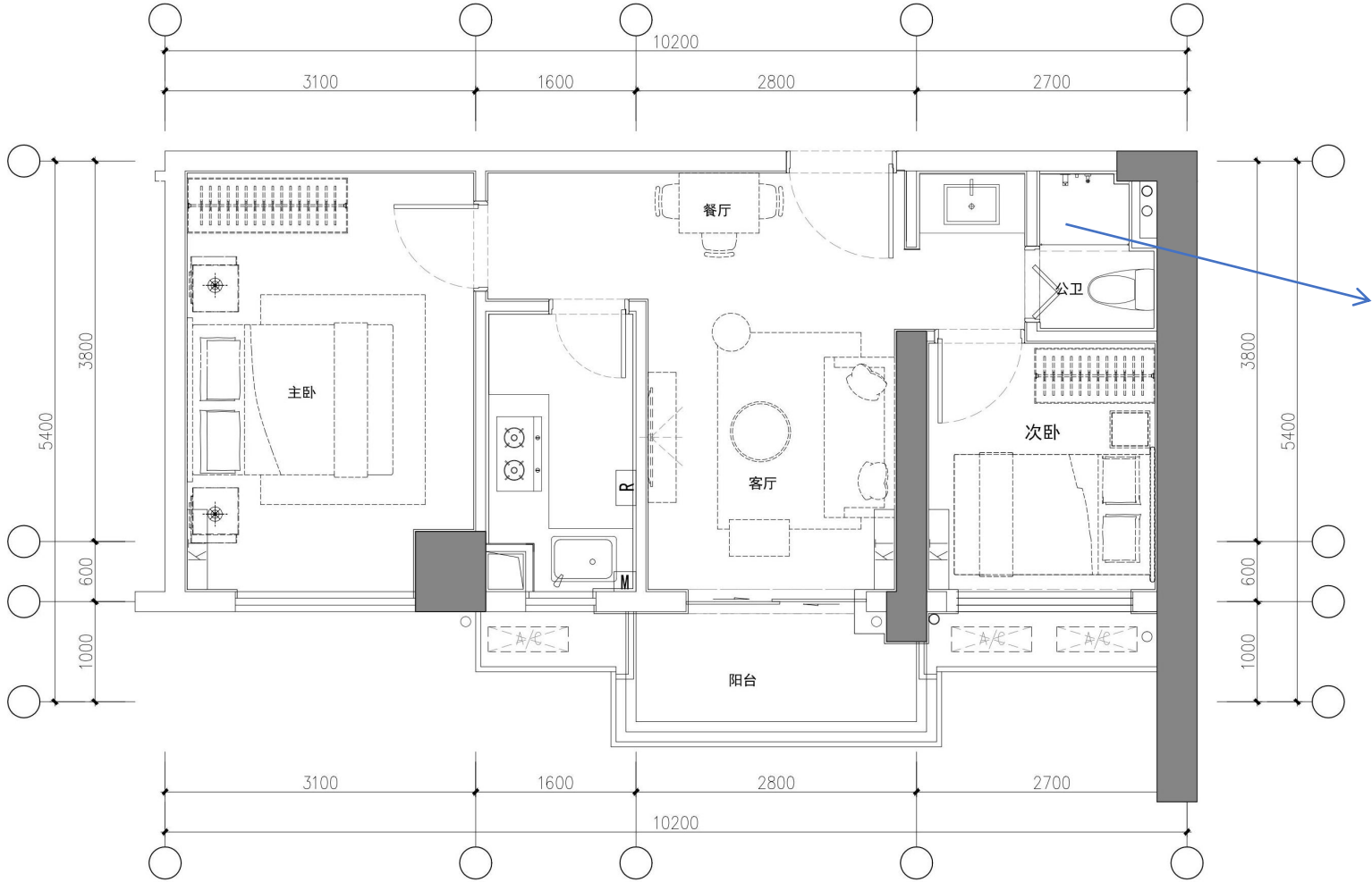
两房一厅标准层平面图
