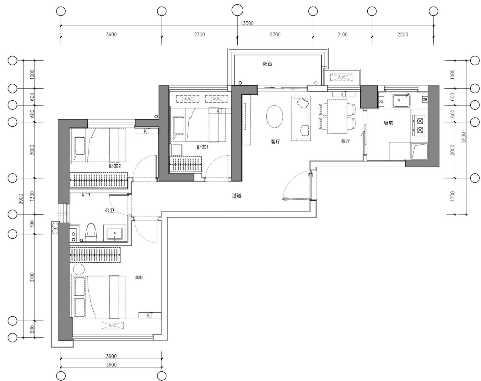
三房一厅标准层平面图
