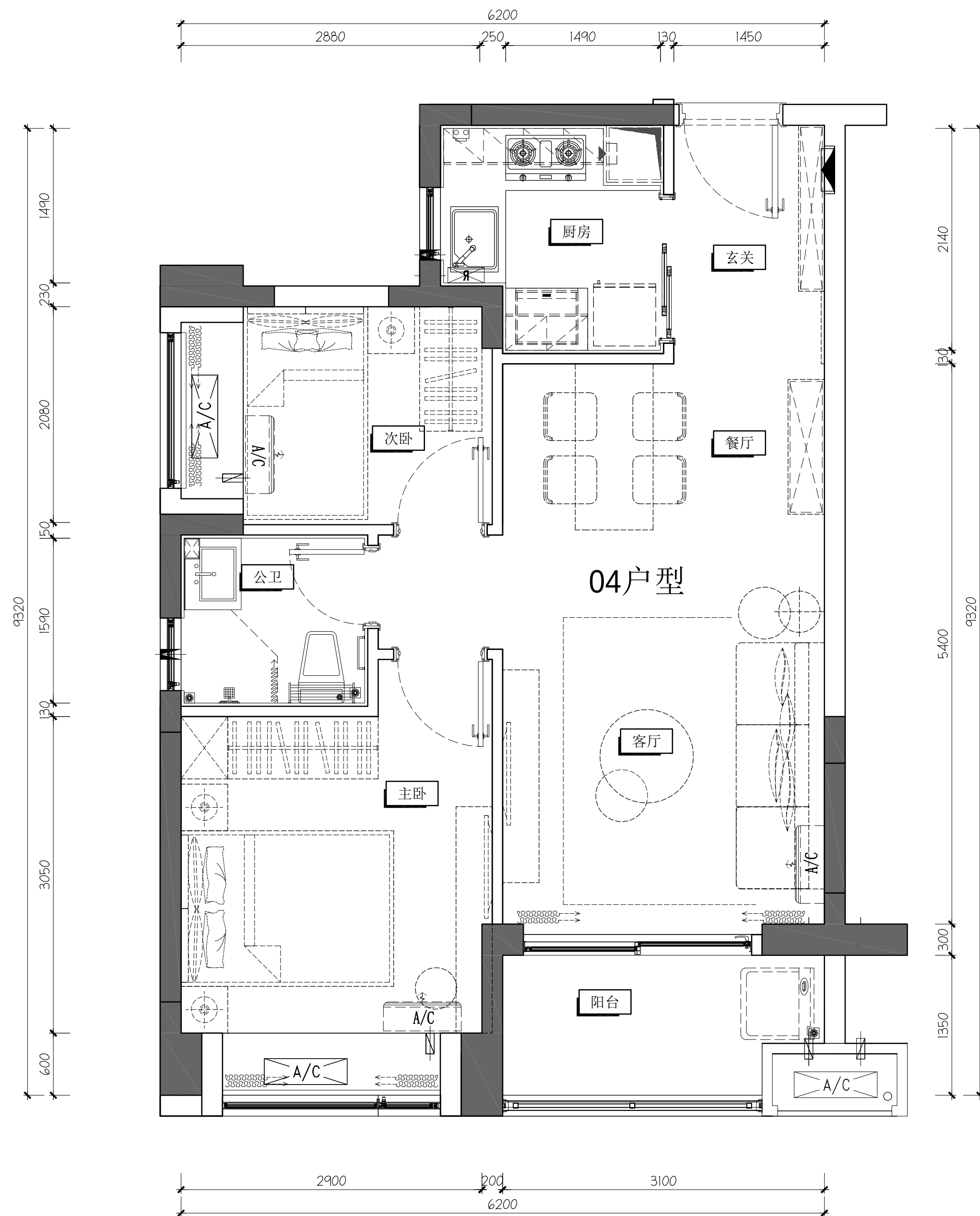
公共租赁住房04户型(两房)平面图 注：面积约66.85平方米
