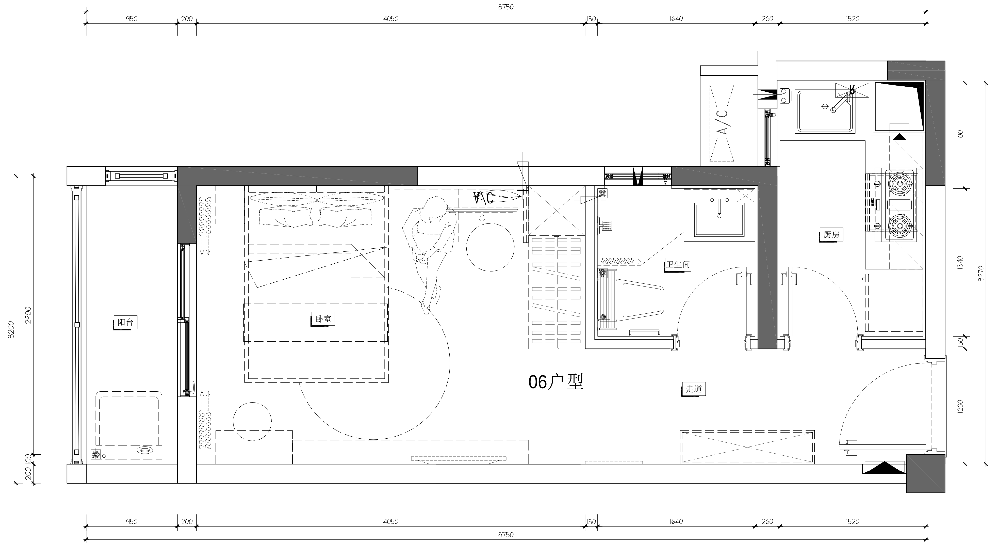
公共租赁住房06户型(一房)平面图 注：面积约36.84平方米
