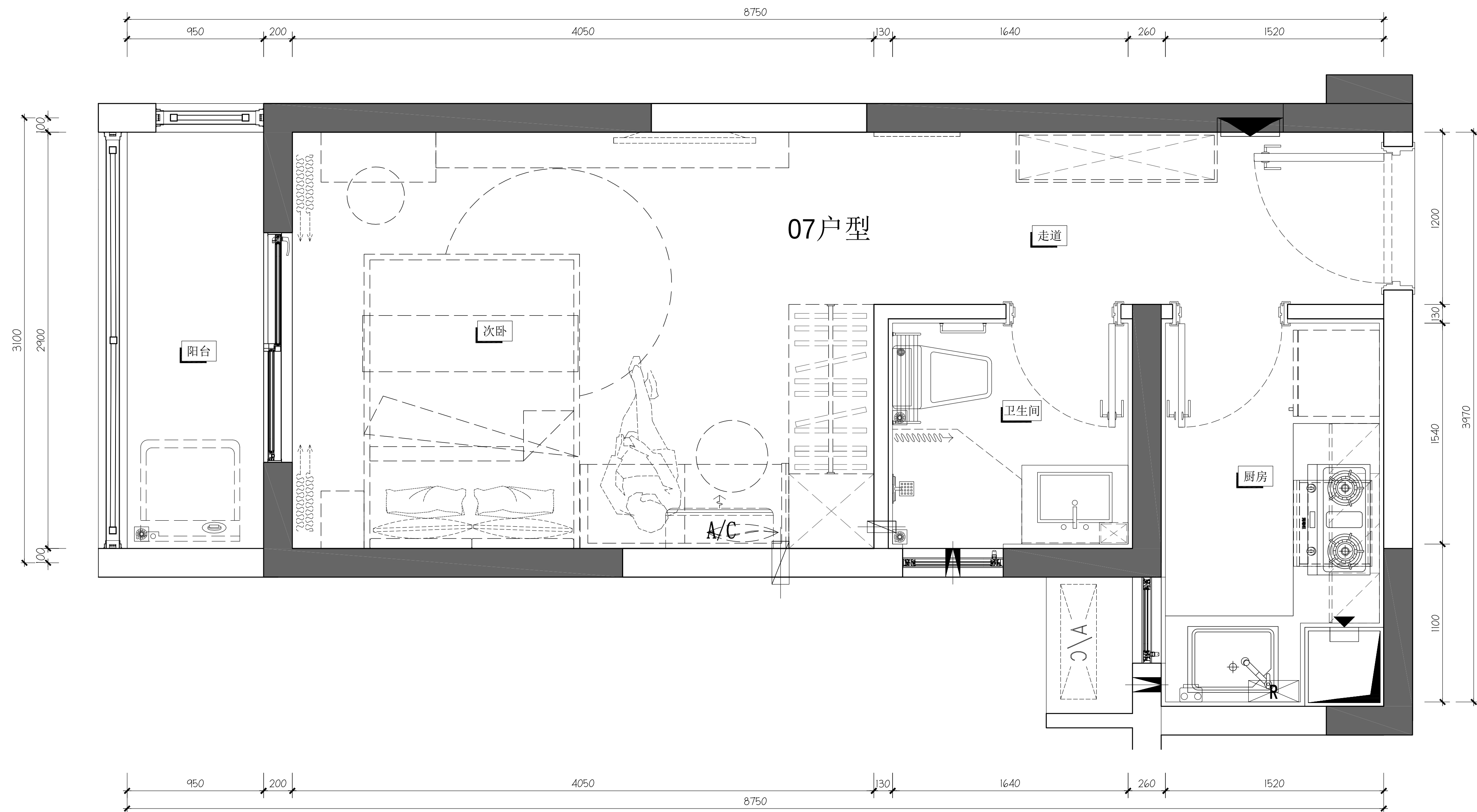
公共租赁住房07户型(一房)平面图 注：面积约36.91平方米
