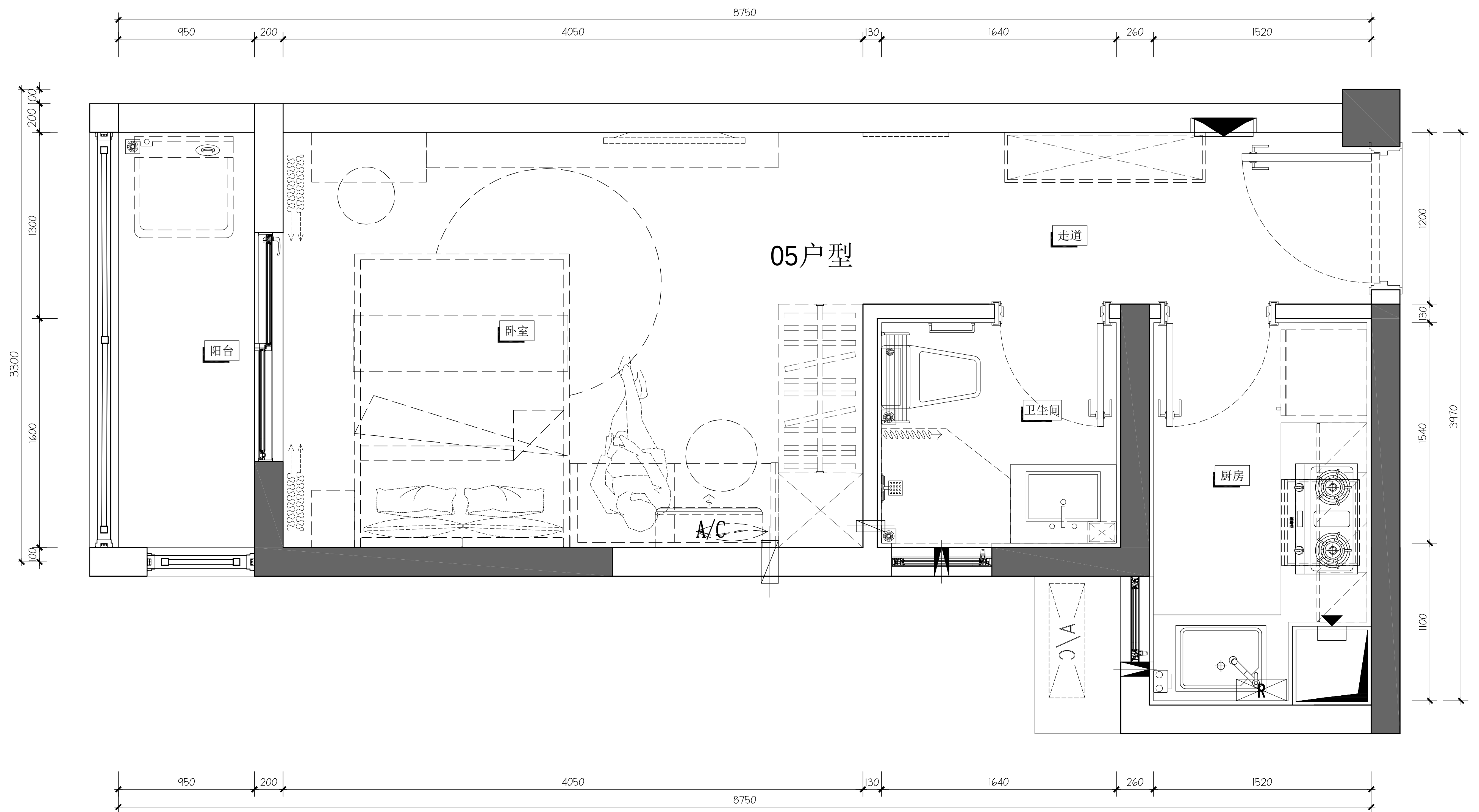
公共租赁住房05户型(一房)平面图 注：面积约36.84平方米
