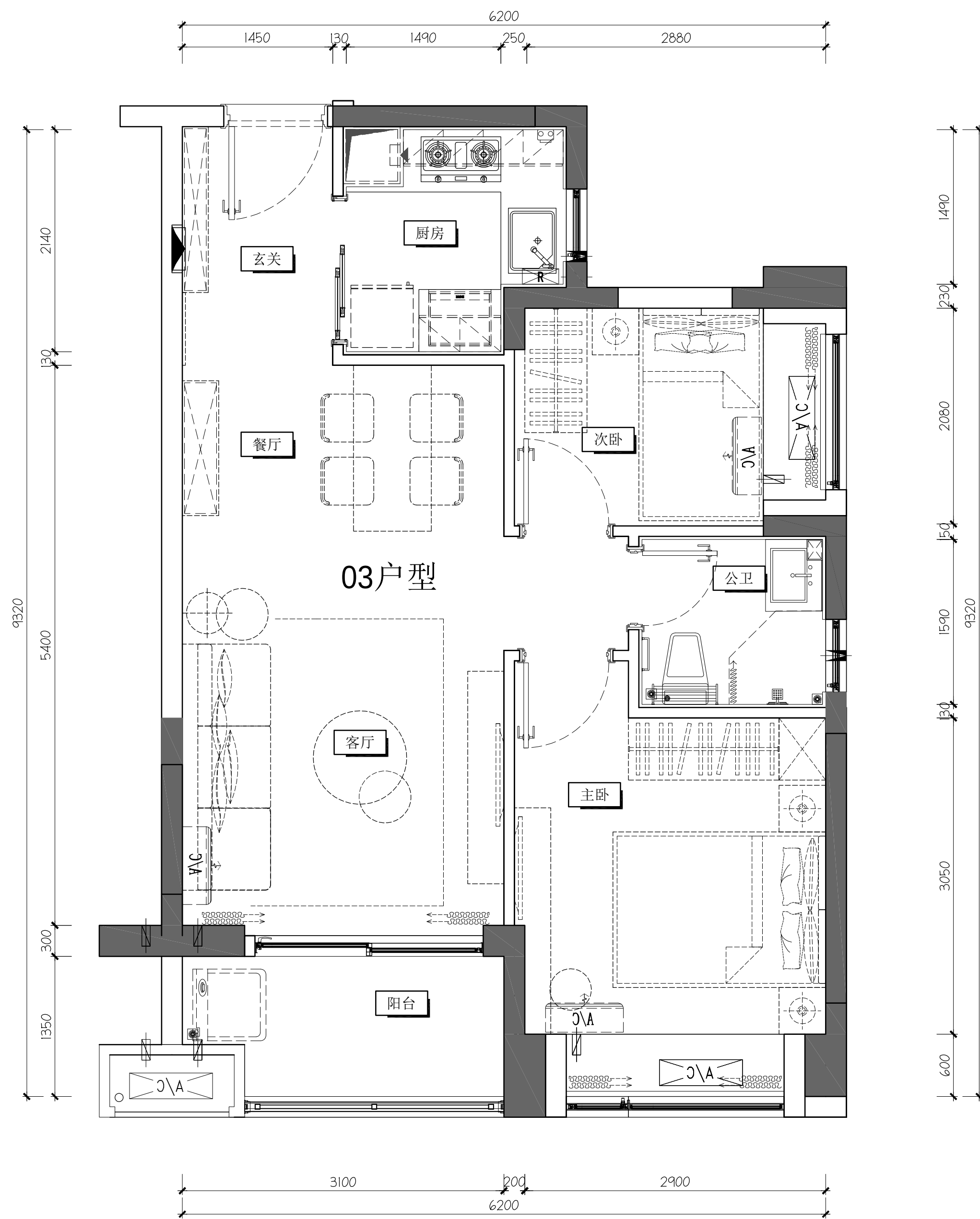
公共租赁住房03户型(两房)平面图 注：面积约66.85平方米
