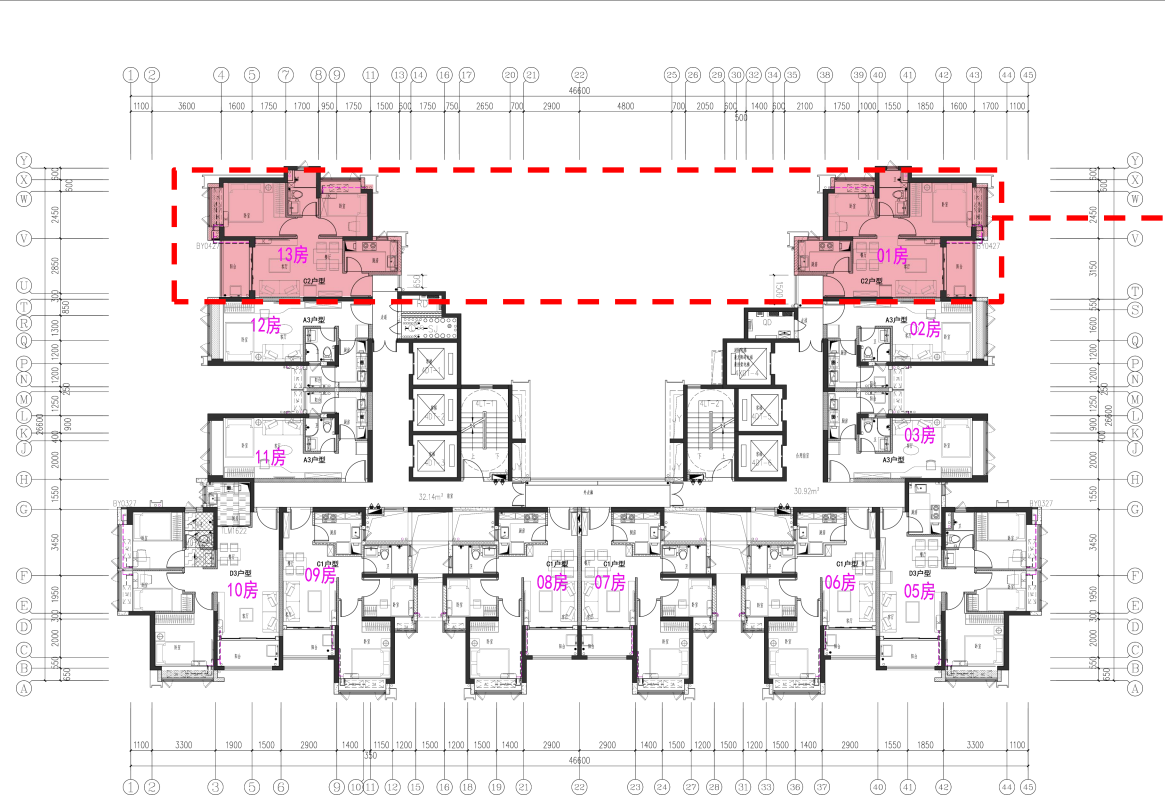
标准层平面图 注：建筑面积约67m²
