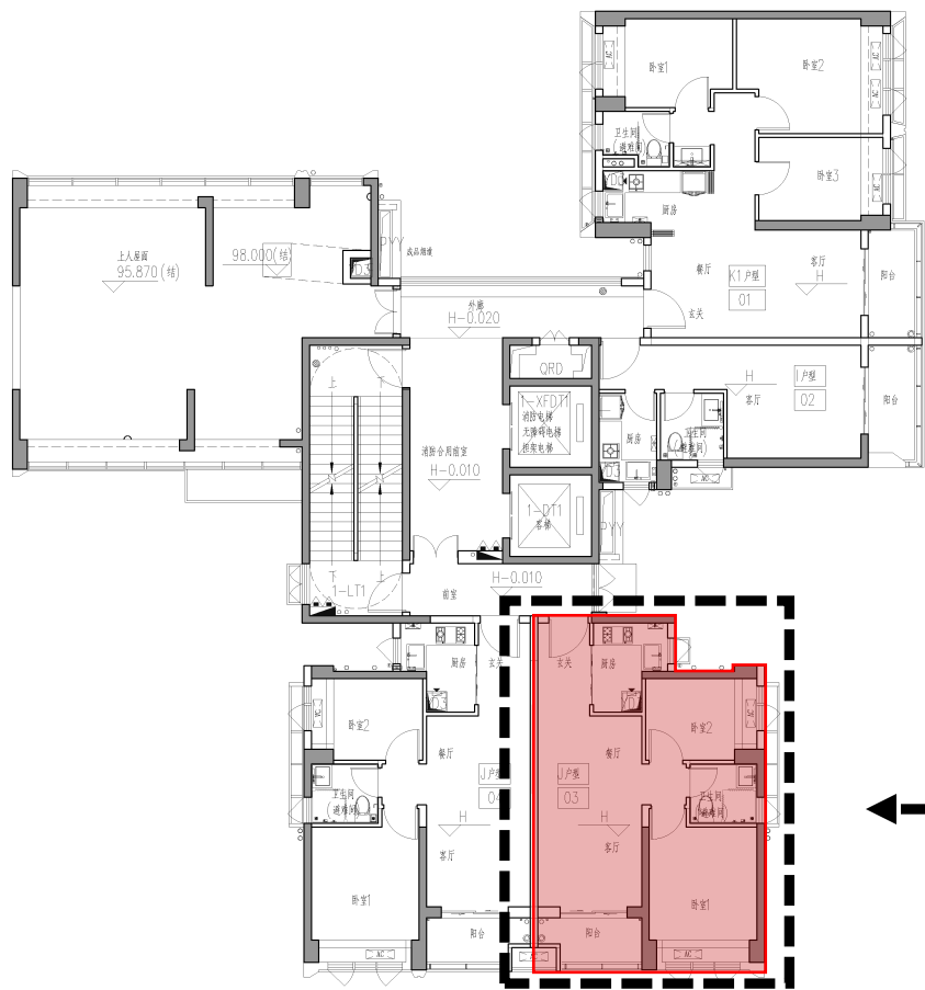
31层平面图
