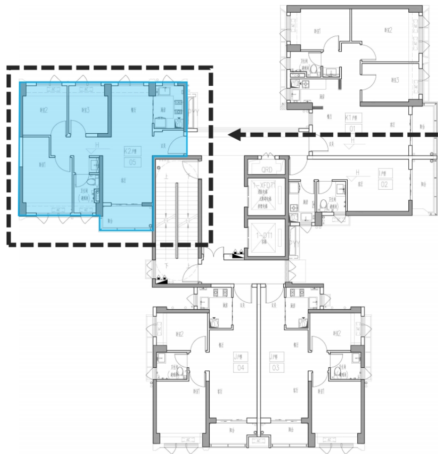
3~30层平面图
