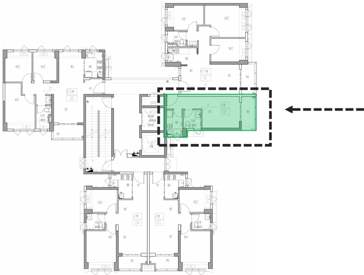
3~30层平面图
