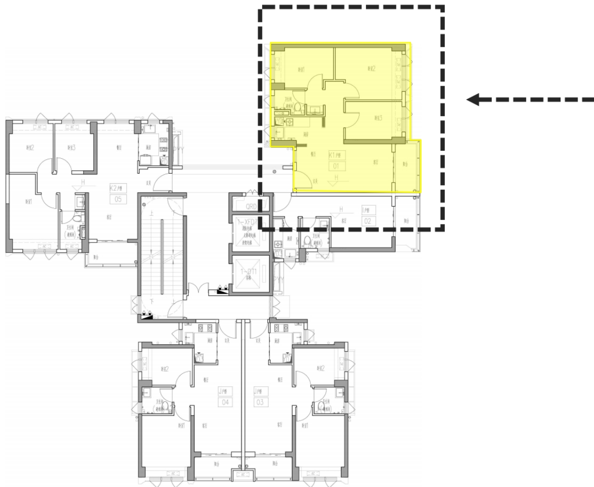
3~30层平面图
