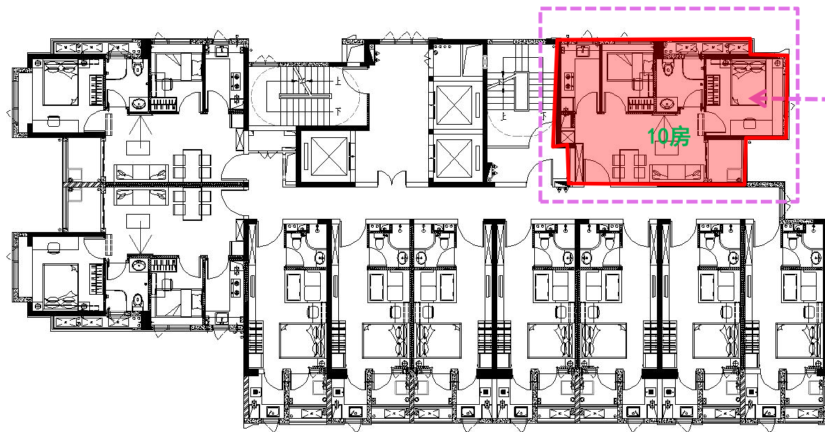
A2户型 10房 7~23层平面位置索引示意图 注：建筑面积约64平方米
