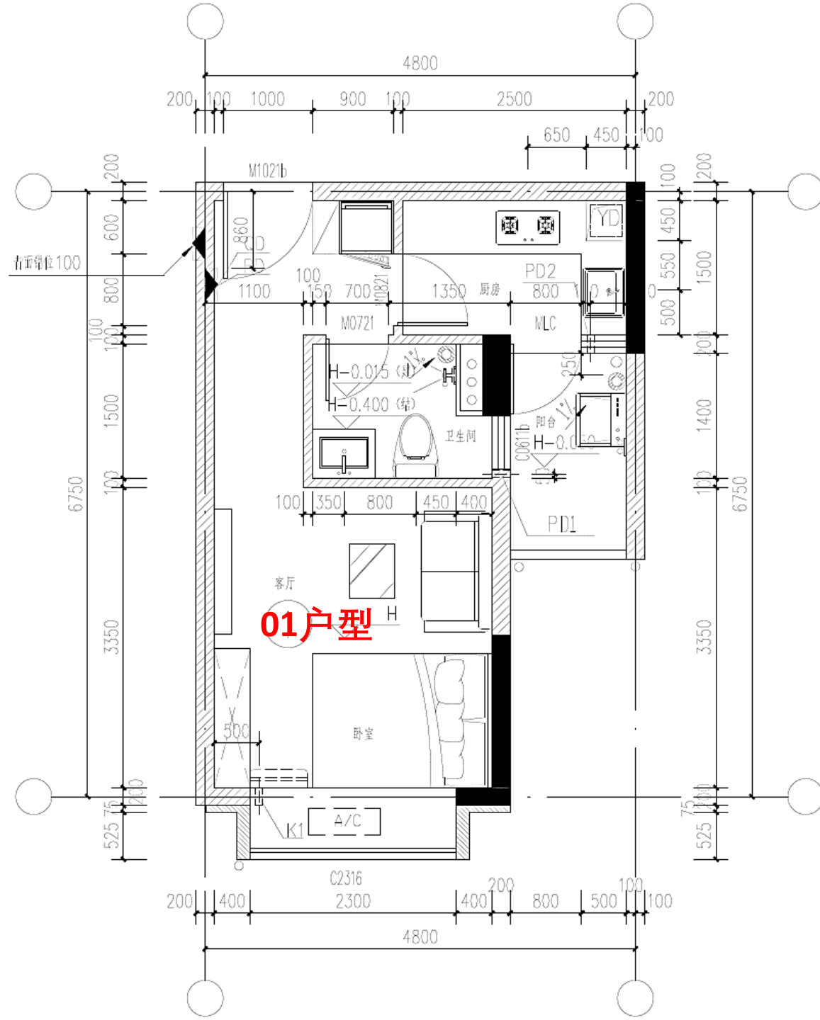
一房标准层平面图
